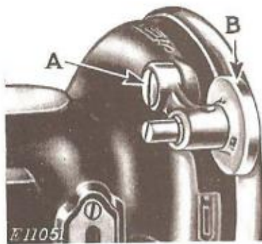
FIG. 30. BOBBIN WINDER
