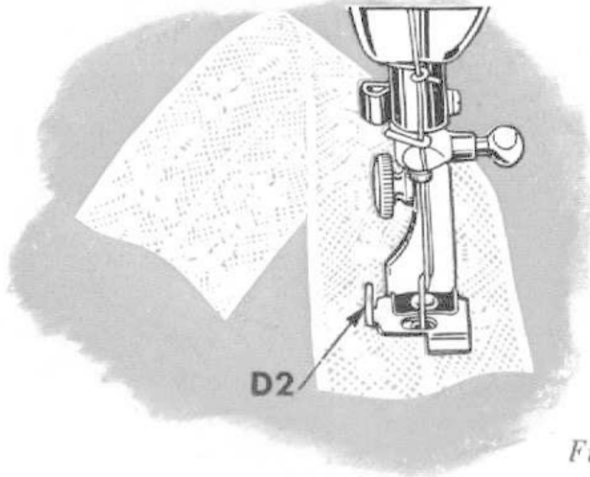
Fig. 52. The Edge Stitcher
